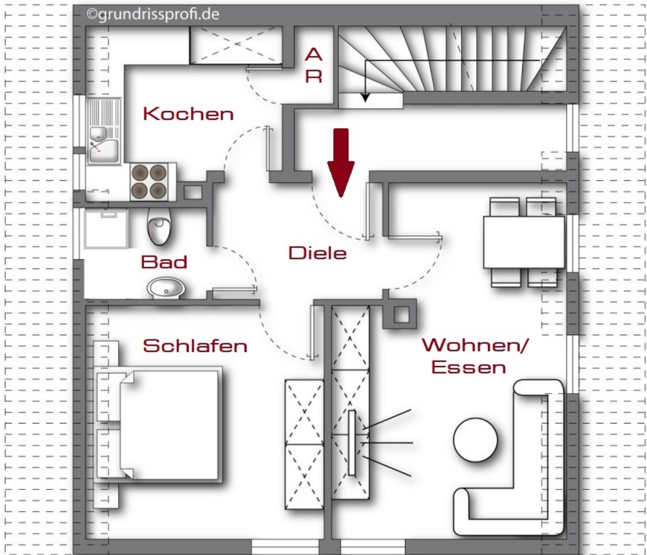
2. Obergeschoss = Dachgeschoss
